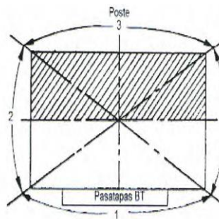
Figura 2. Designación de segmentos para transformadores rectangulares
