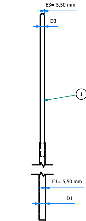
VISTA FRONTAL ESC: ( 1 : 50 )
