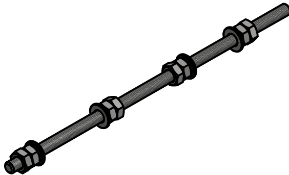
VISTA ISOMETRICA ESC: ( 1 : 5 )
