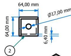
VISTA DE PERFIL ESC: ( 1 : 7.5 )
