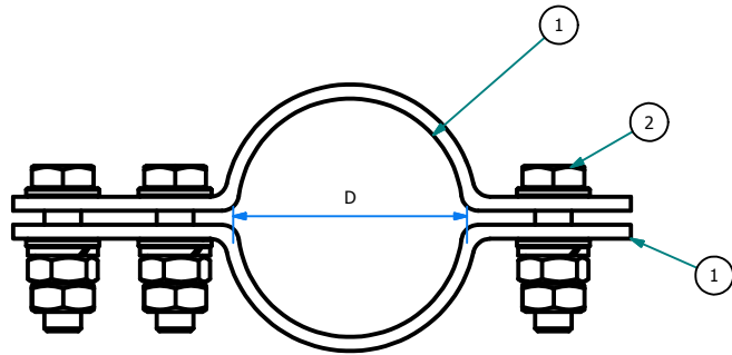
VISTA FRONTAL ESC: 1 : 3
