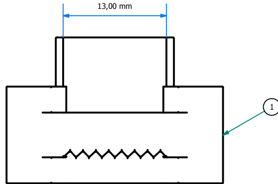
VISTA FRONTAL ESC: 2 : 1
