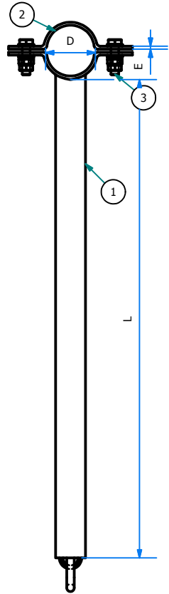
VISTA FRONTAL ESC: 1 : 9
