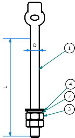
VISTA FRONTAL ESC: 1 : 4
