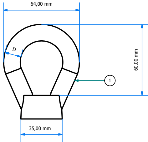
VISTA FRONTAL ESC: 1 : 2
