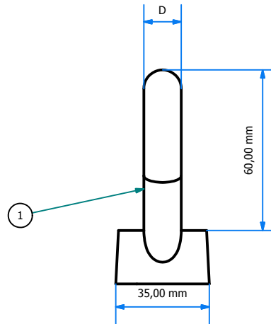
VISTA DE PERFIL ESC: 1 : 2
