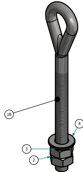
VISTA ISOMETRICA ESC: 1 : 2.5
