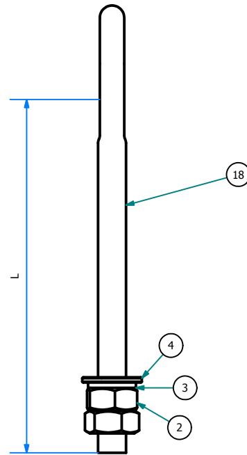
VISTA DE PERFIL ESC: 1 : 3
