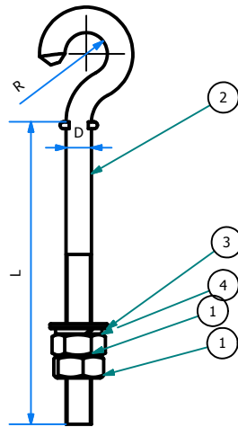
VISTA FRONTAL ESC: 1 : 4
