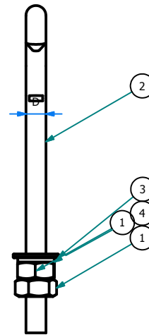
VISTA DE PERFIL ESC: 1 : 4
