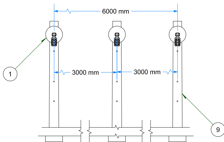
VISTA FRONTAL ESC: 1 / 35
