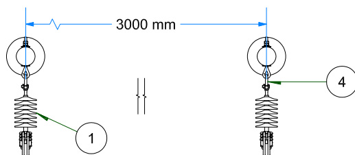
VISTA DE PLANTA ESC: 1 / 35
