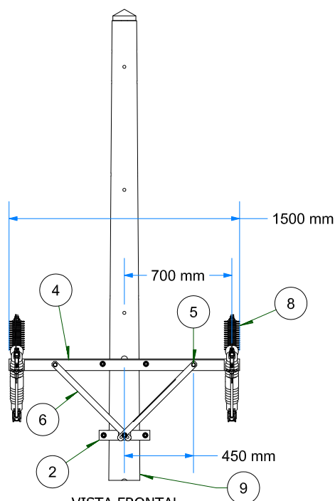
VISTA FRONTAL ESC: 1 / 35
