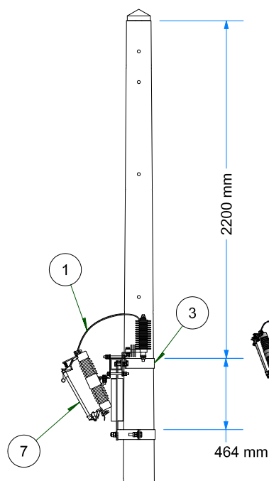
VISTA DE PERFIL ESC: 1 / 35
