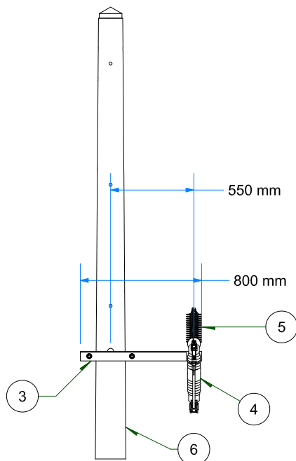
VISTA FRONTAL ESC: 1 / 35
