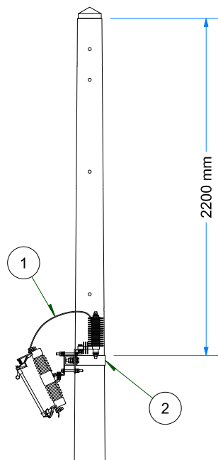
VISTA DE PERFIL ESC: 1 / 35
