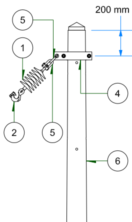
VISTA FRONTAL ESC: 1 / 35
