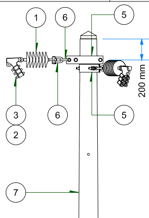
VISTA DE PERFIL ESC: 1 / 35
