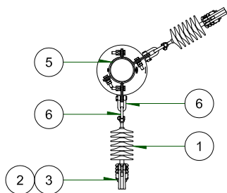
VISTA DE PLANTA ESC: 1 / 35
