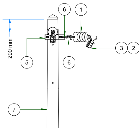
VISTA FRONTAL ESC: 1 / 35
