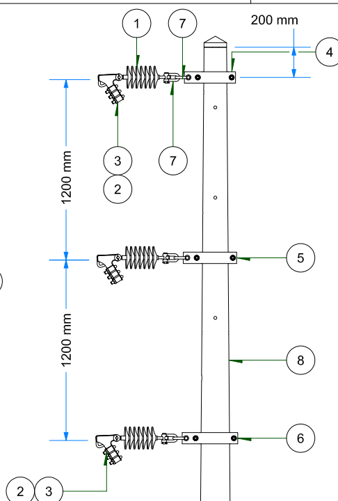
VISTA DE PERFIL ESC: 1 / 35
