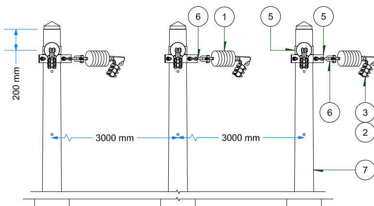
VISTA DE FRENTE ESC: 1 / 35
