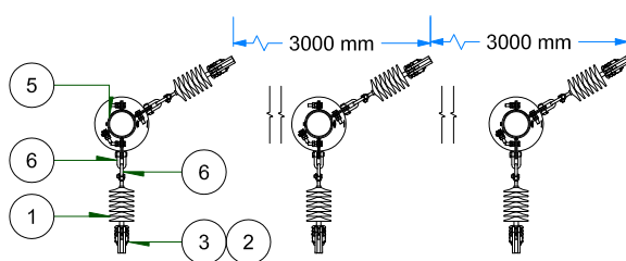
VISTA DE PLANTA
