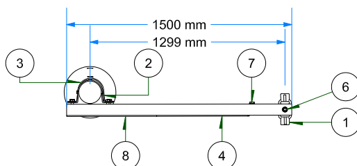
VISTA DE PLANTA ESC: 1 / 35
