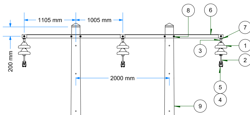
VISTA FRONTAL ESC: 1 / 50
