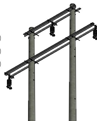
VISTA ISOMETRICA ESC: 1 / 75
