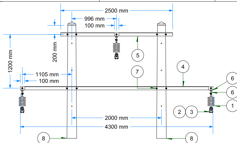
VISTA FRONTAL ESC: 1 / 50
