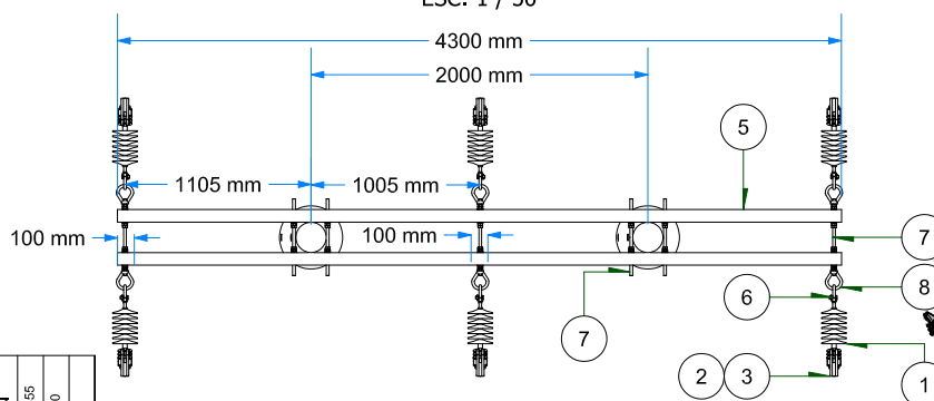
VISTA DE PLANTA ESC: 1 / 50
