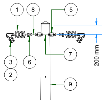
VISTA DE PERFIL ESC: 1 / 50
