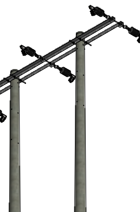
VISTA ISOMETRICA ESC: 1 / 75
