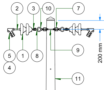
VISTA DE PERFIL ESC: 1 / 50
