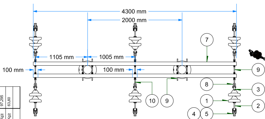
VISTA DE PLANTA ESC: 1 / 50
