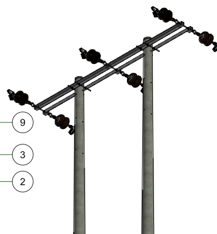
VISTA ISOMETRICA ESC: 1 / 75
