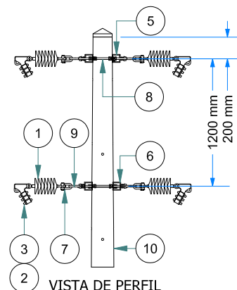
VISTA DE PERFIL ESC: 1 / 50
