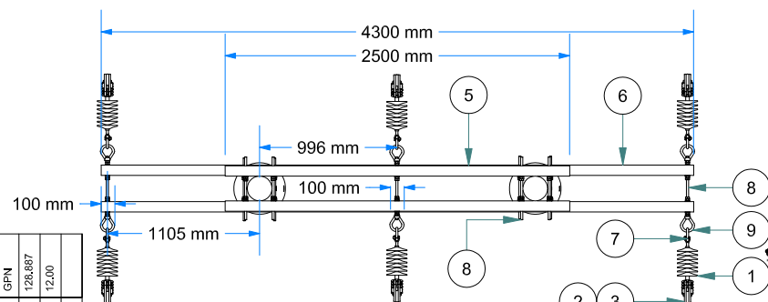
VISTA DE PLANTA ESC: 1 / 50
