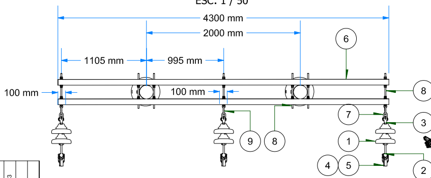
VISTA DE PLANTA ESC: 1 / 50
