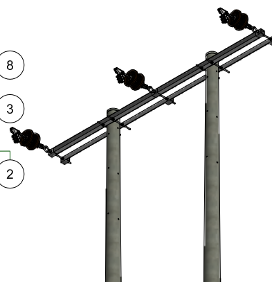
VISTA ISOMETRICA ESC: 1 / 75
