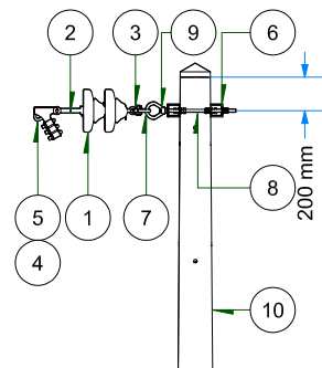
VISTA DE PERFIL ESC: 1 / 50
