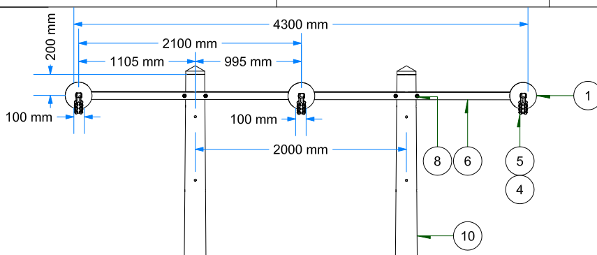
VISTA FRONTAL ESC: 1 / 50
