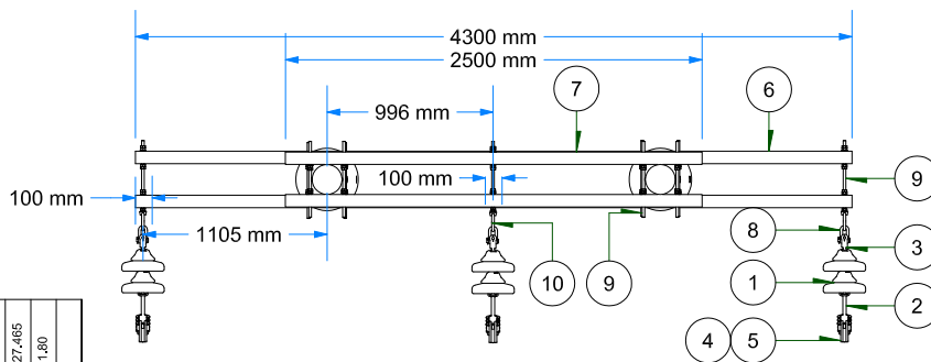
VISTA DE PLANTA ESC: 1 / 50
