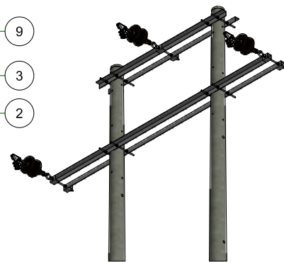
VISTA ISOMETRICA ESC: 1 / 75
