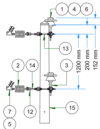
VISTA DE PERFIL ESC: 1 / 50
