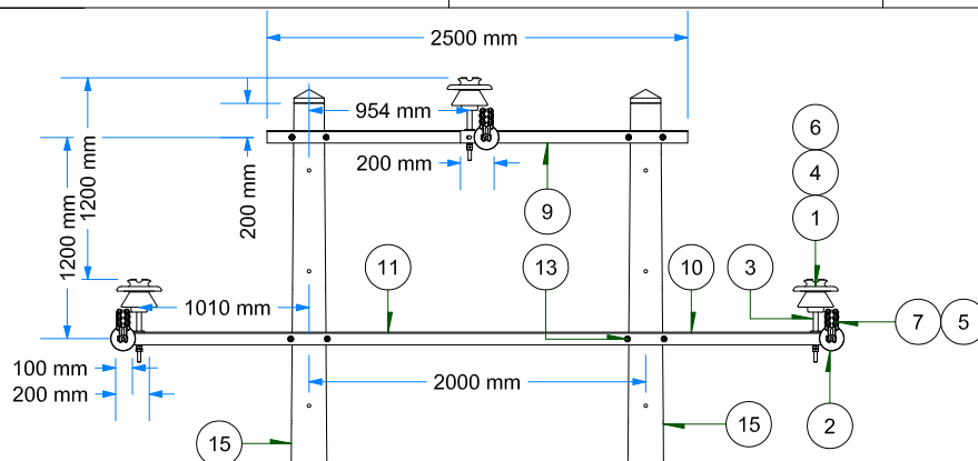
VISTA FRONTAL ESC: 1 / 50
