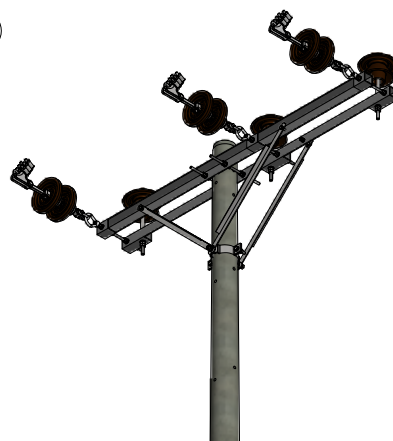
VISTA ISOMETRICA ESC: 1 / 50
