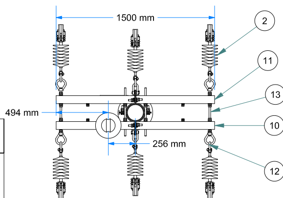
VISTA DE PLANTA ESC: 1 / 35
