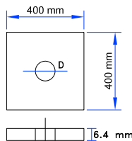
DETALLE DE LA PLANCHA
