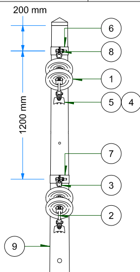
VISTA FRONTAL ESC: 1 / 35
