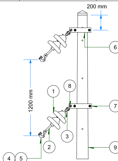
VISTA DE PERFIL ESC: 1 / 35
