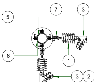
VISTA FRONTAL ESC: 1 / 35
