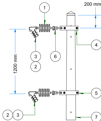
VISTA DE PERFIL ESC: 1 / 35
