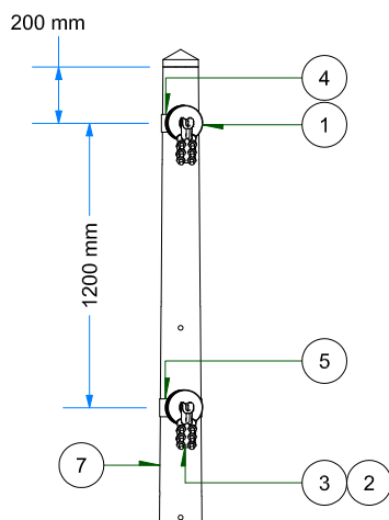
VISTA FRONTAL ESC: 1 / 35
