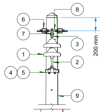
VISTA DE PERFIL ESC: 1 / 35
