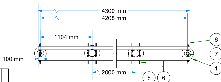
VISTA DE PLANTA ESC: 1 / 50
