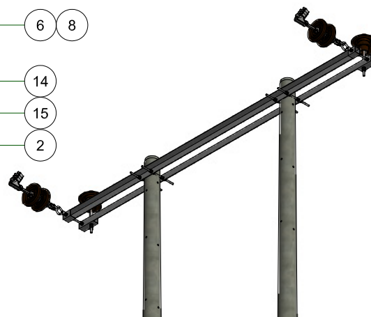
VISTA ISOMETRICA ESC: 1 / 50
