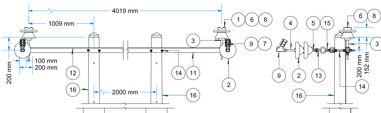
VISTA FRONTAL ESC: 1 / 35
