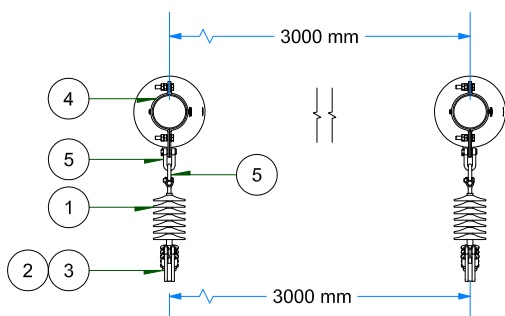
VISTA DE PLANTA ESC: 1 / 35
