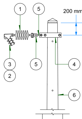
VISTA DE PERFIL ESC: 1 / 35
