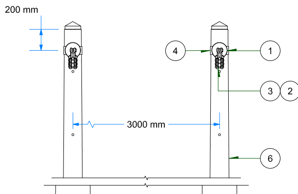
VISTA DE FRENTE ESC: 1 / 35
