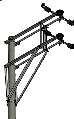
VISTA ISOMETRICA ESC: 1 / 75
