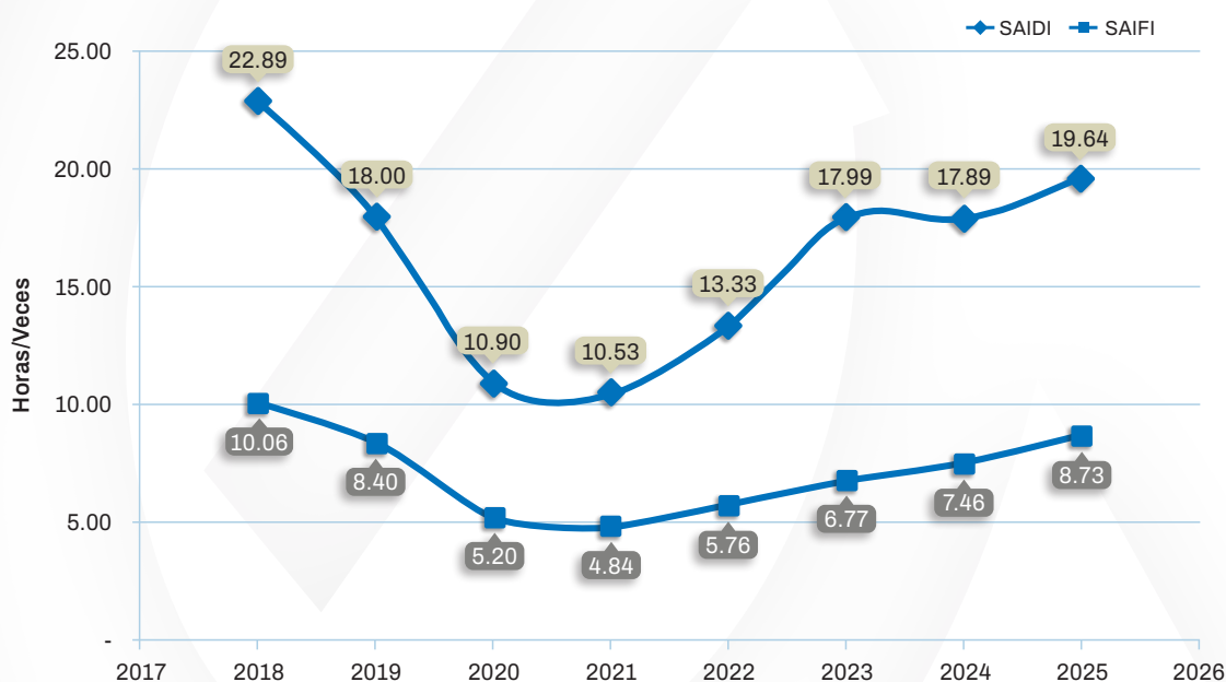
Evolución Indicadores SAIDI y SAIFI
